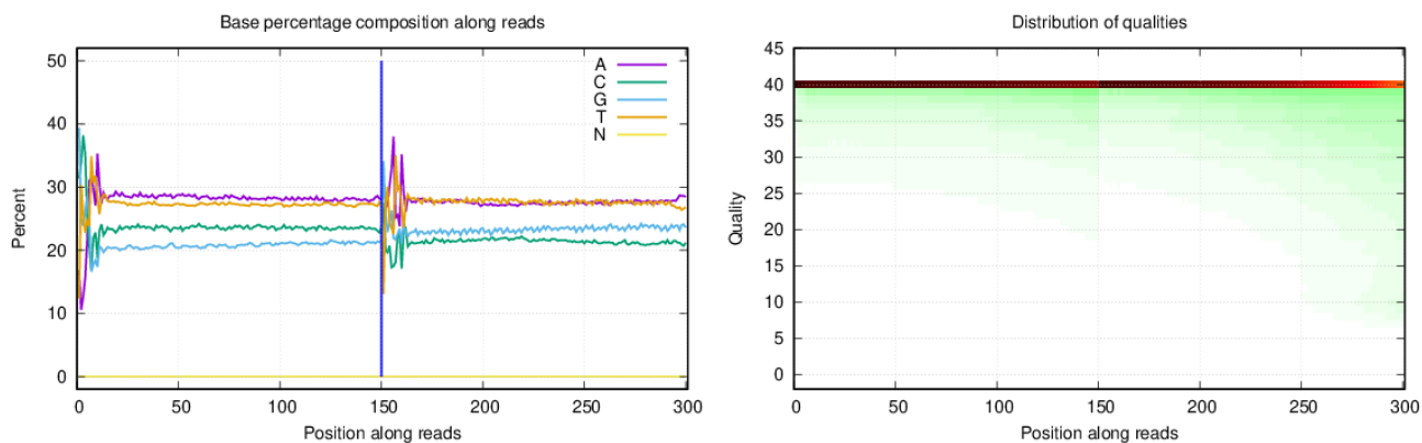
图9 5单碱基组分分布图和单碱基质量分布图
