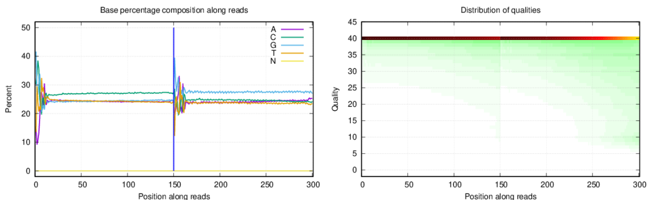
图12 11单碱基组分分布图和单碱基质量分布图
