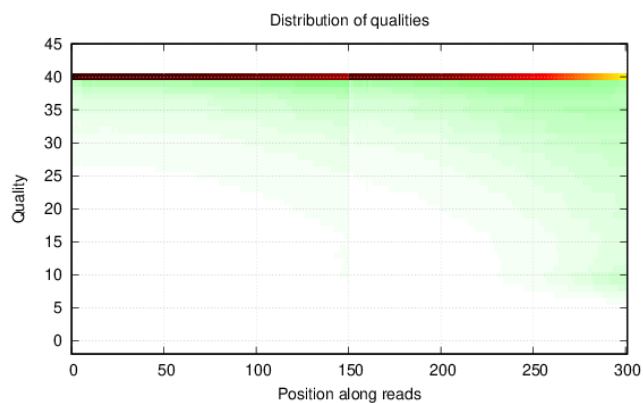
图6 10单碱基组分分布图和单碱基质量分布图
