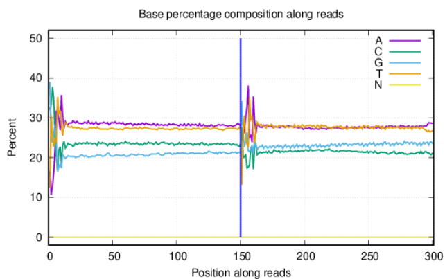
图8 4单碱基组分分布图和单碱基质量分布图
