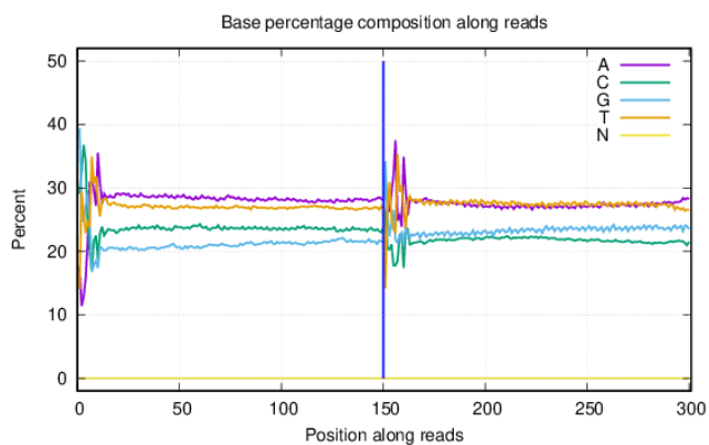
图3 3单碱基组分分布图和单碱基质量分布图
