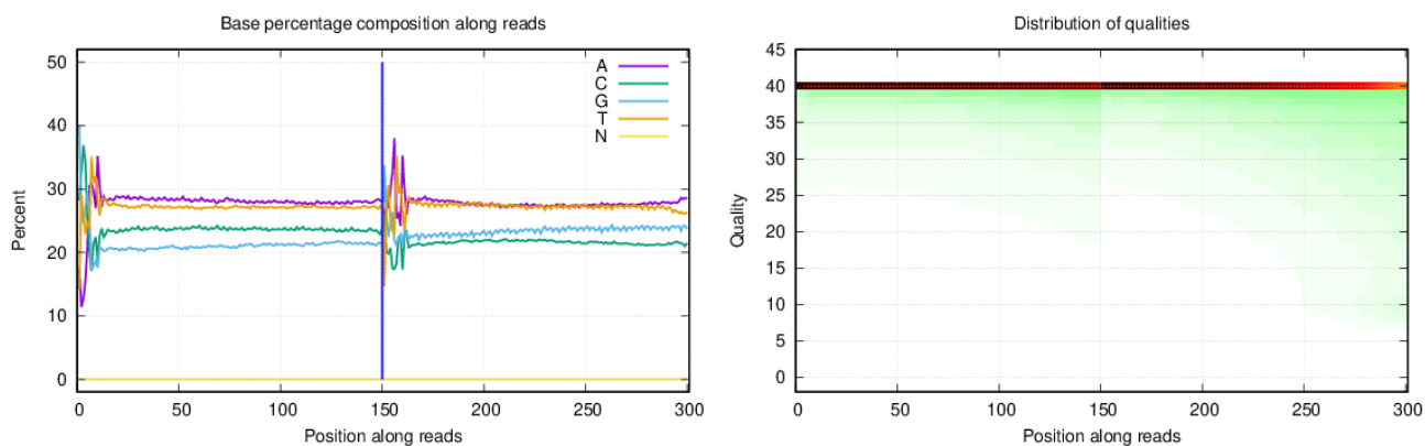
图10 7单碱基组分分布图和单碱基质量分布图
