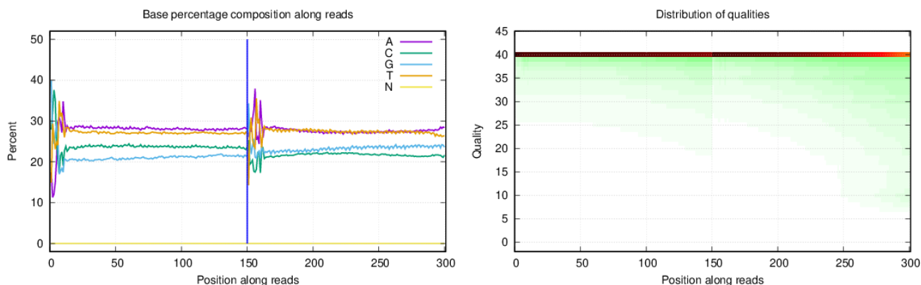
图1 8单碱基组分分布图和单碱基质量分布图
