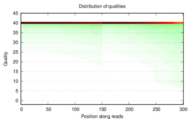
图7 9单碱基组分分布图和单碱基质量分布图
