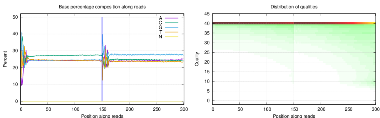
图2 12单碱基组分分布图和单碱基质量分布图
