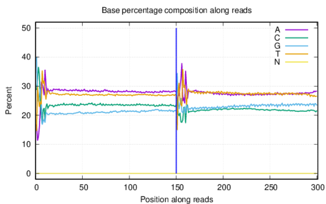
图5 2单碱基组分分布图和单碱基质量分布图
