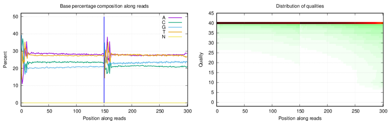
图11 6单碱基组分分布图和单碱基质量分布图
