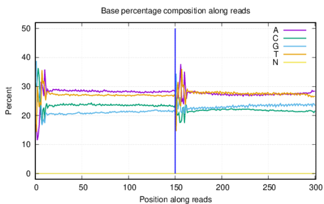
图4 1单碱基组分分布图和单碱基质量分布图
